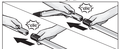
Afb. 3: Opsteken van de verlengpijpen
