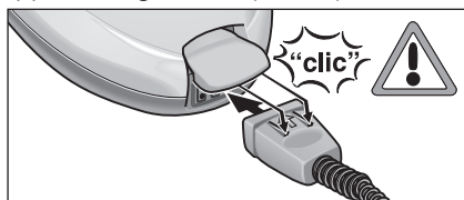
III. 1: Isättning av blockkontakten
